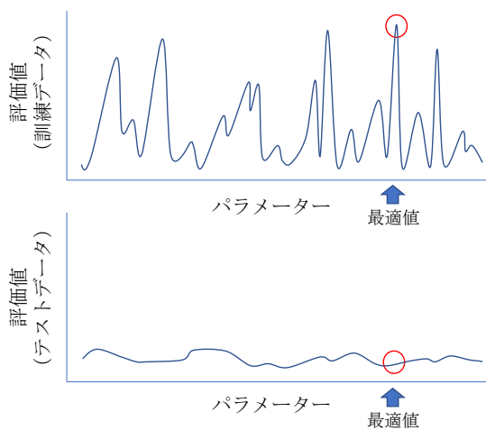
図 1a : 評価関数の形状とモデルの汎用性：急峻な多峰性の場合
