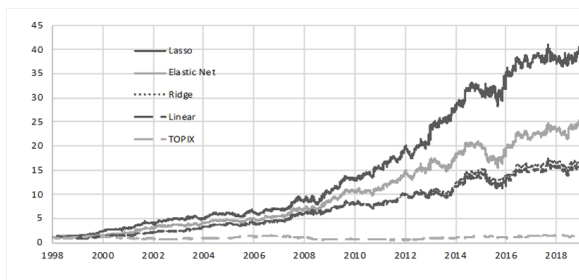
図 3：各モデルの累積リターンの推移
