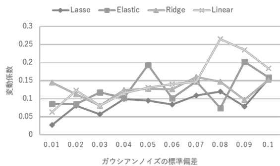
図 5：ノイズ付与時の累積リターンの変動係数
