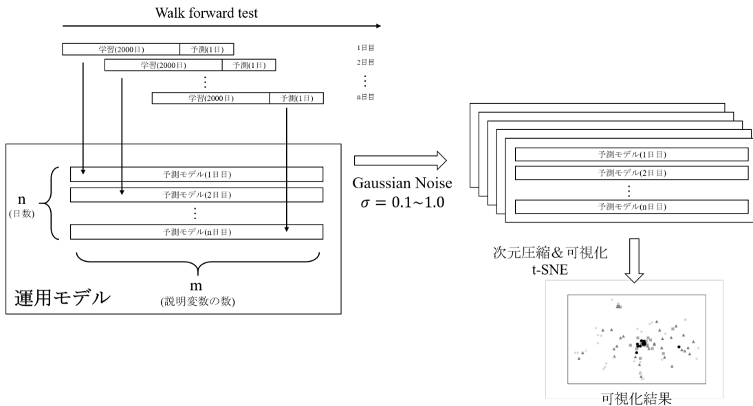
図 2 : モデルの安定性の評価方法
