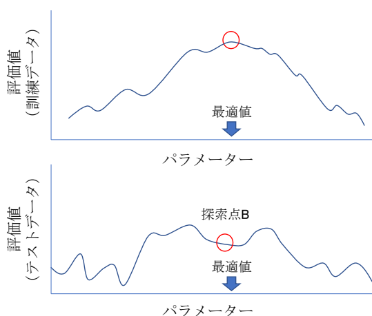
図 1b : 評価関数の形状とモデルの汎用性：緩やかな単峰性の場合
